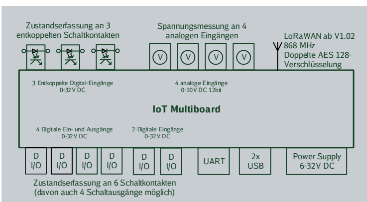
Abbildung 2: Blockschaltbild IoT Multiboard
