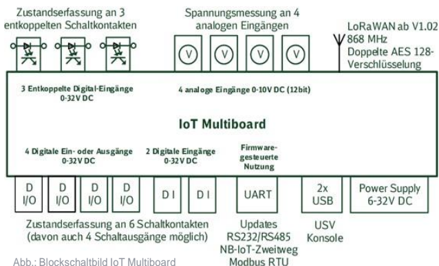
Abb.: Blockschaltbild IoT Multiboard
